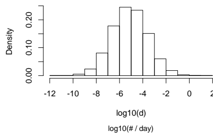
Histogram of log 10 (d)
