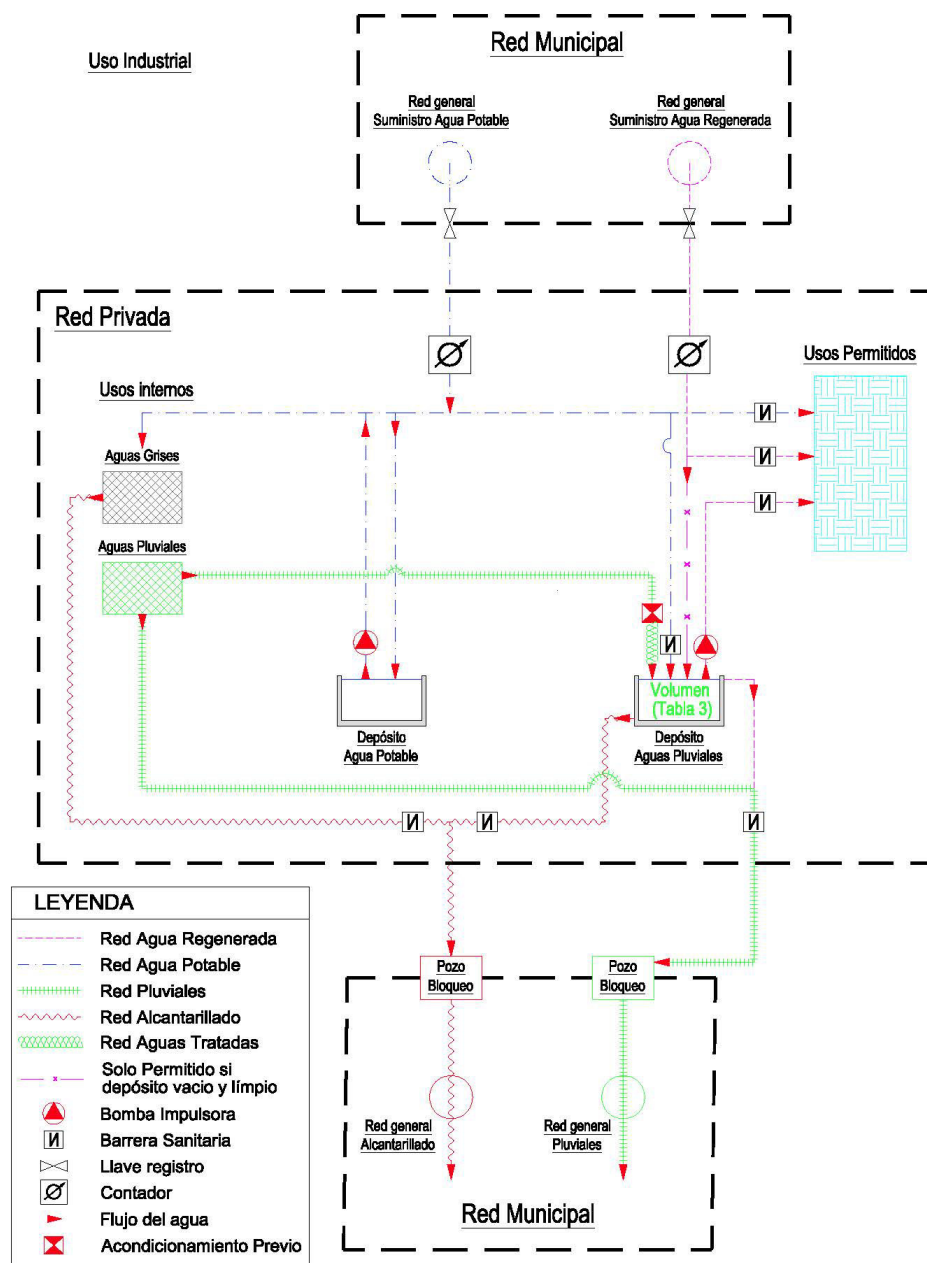
FIGURA 2. ESQUEMA INSTALACIÓN AGUAS REGENERADAS Y PLUVIALES
