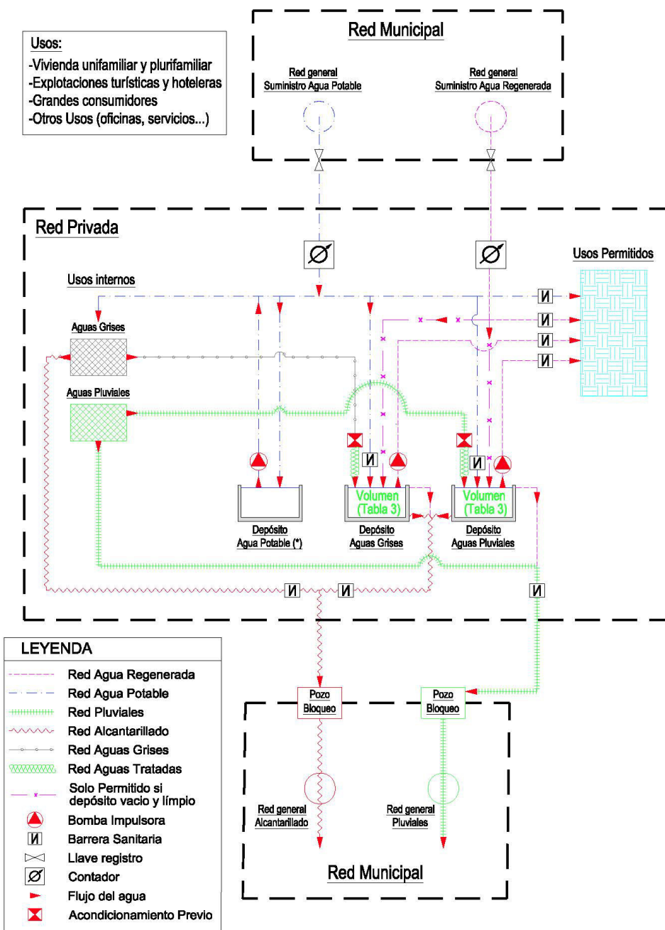
FIGURA 1. ESQUEMA INSTALACIÓN AGUAS GRISES, REGENERADAS Y PLUVIALES
